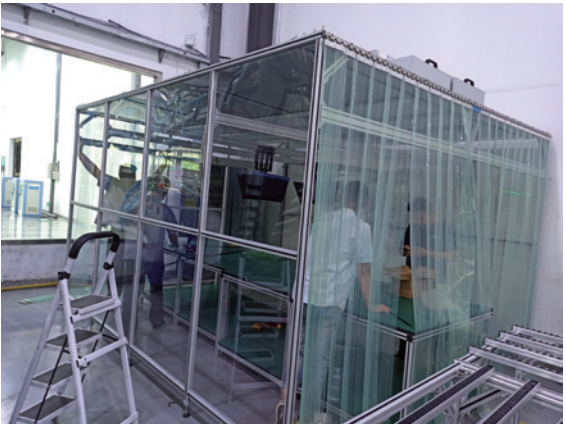
◎ 防弧光焊接房施工
